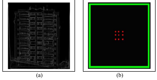
Şekil 4: Bir bina yüzü için oluşan (a) gradyan görüntü ve (b) başlangıç işaretçi piksel şablonu
